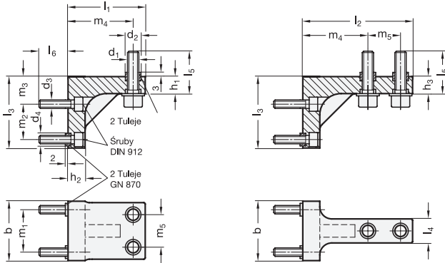
Przykłady montażu
